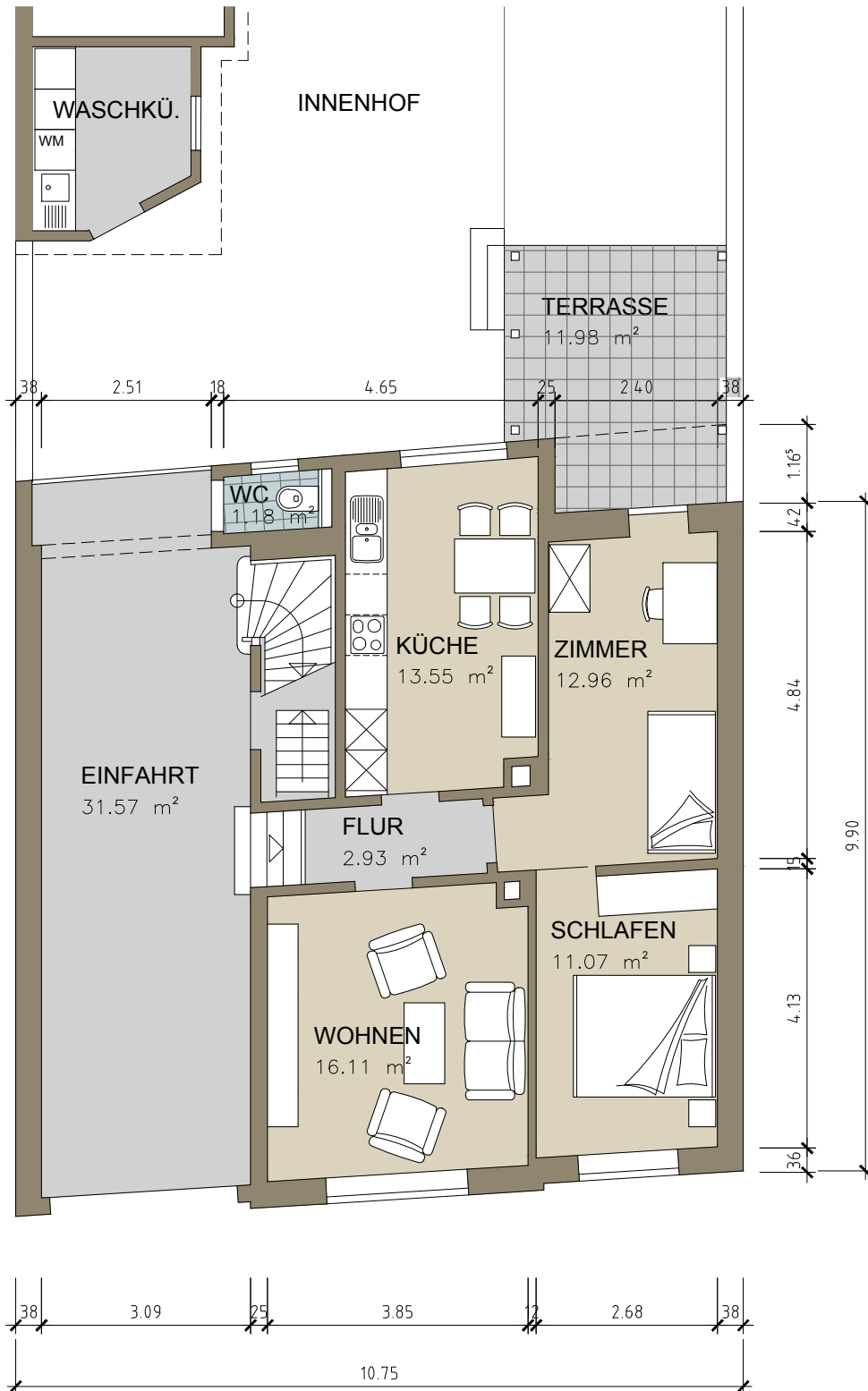
ERDGESCHOSS 1:100
