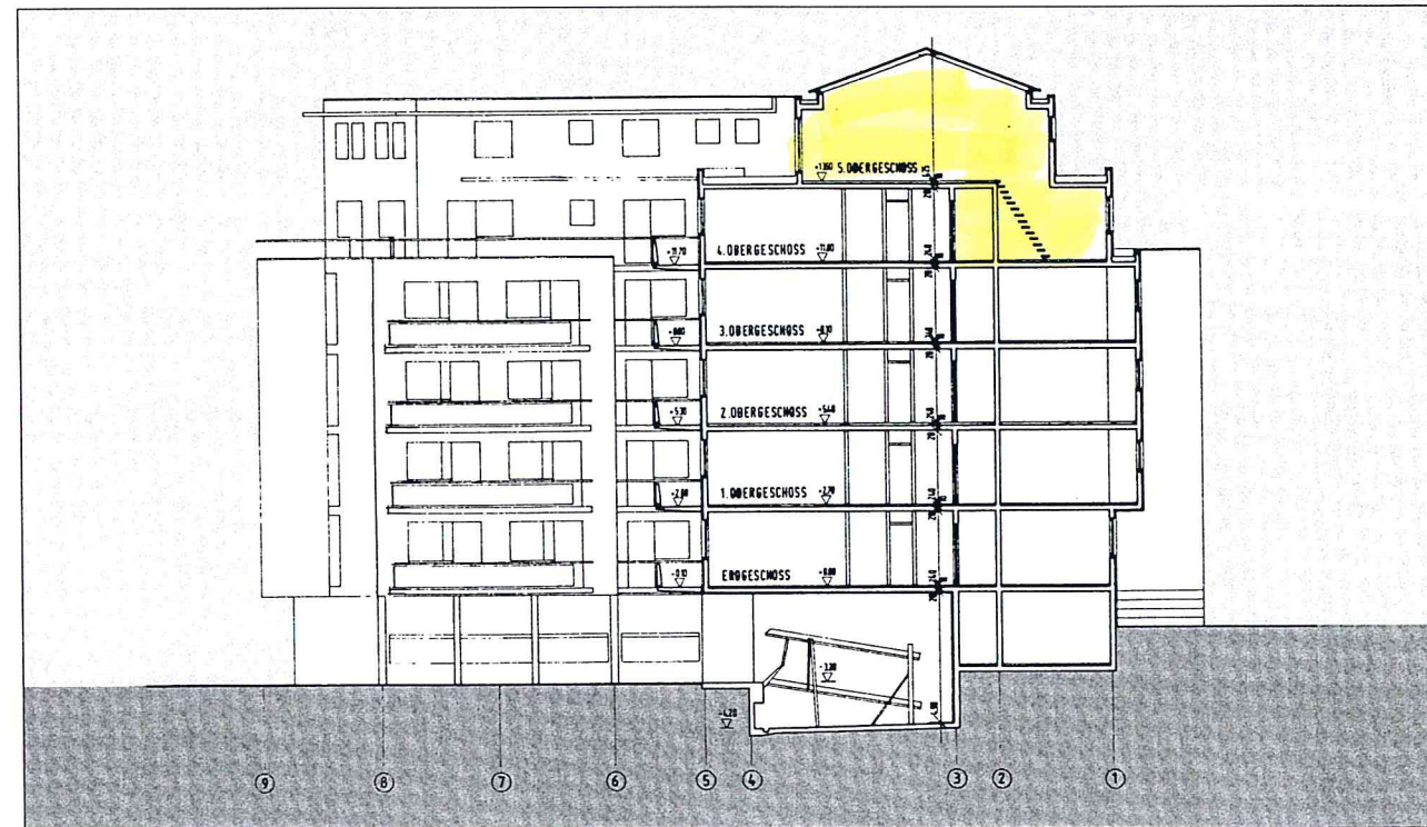
Ansicht Südost/Schnitt
